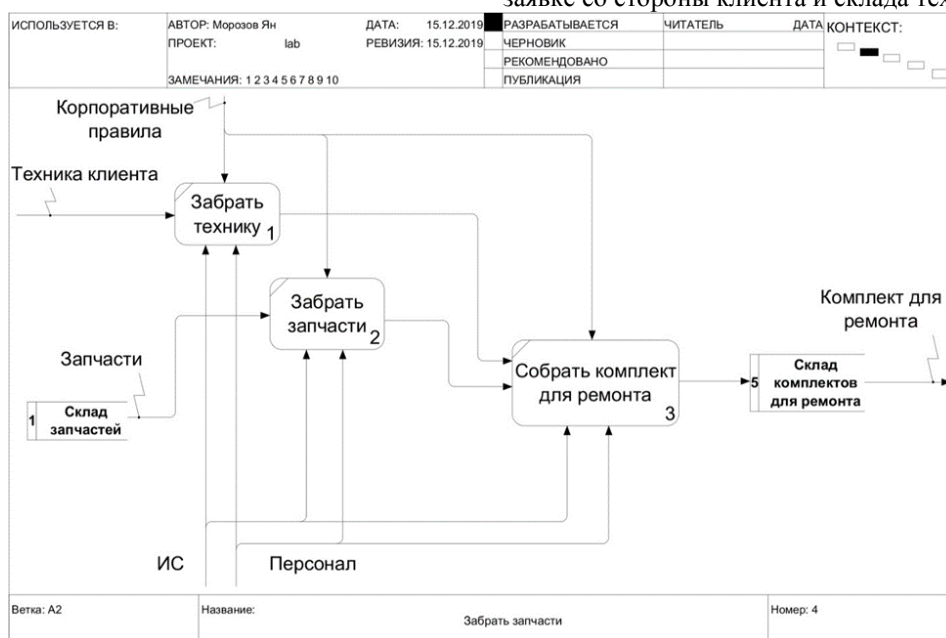
Рисунок 4 – Декомпозиция блока A2
