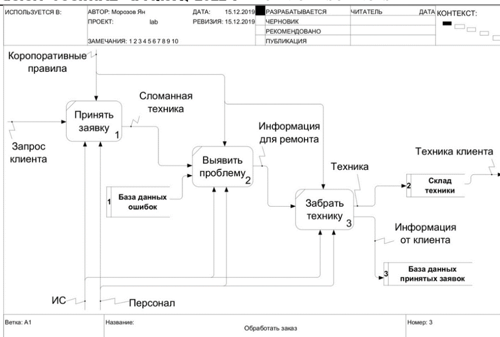
Рисунок 3 – Декомпозиция блока A1
