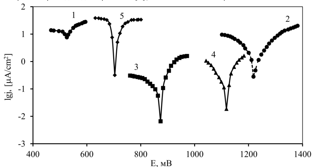
Рис. 1 – Поляризаційні залежності сталі без покриття (1), із покриттям Cr-CrOx, (2), Cr-CrOx-TiOy, (3), Cr-CrOx-AlxOy (4), Cr-CrOx-SiOy, (5).
