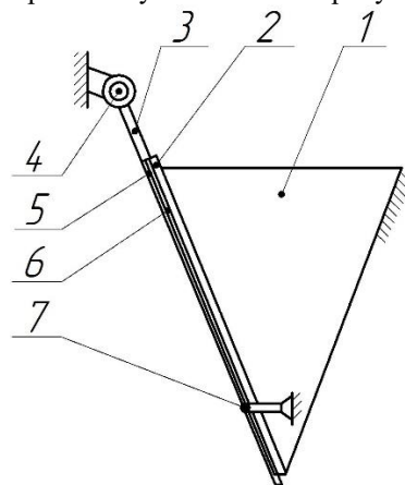
Рисунок 1. Схема вібраційного висівного апарату для посіву дрібнонасінних культур
