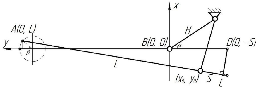
Рисунок 2. Схема роботи висівного апарату (повернуто)
